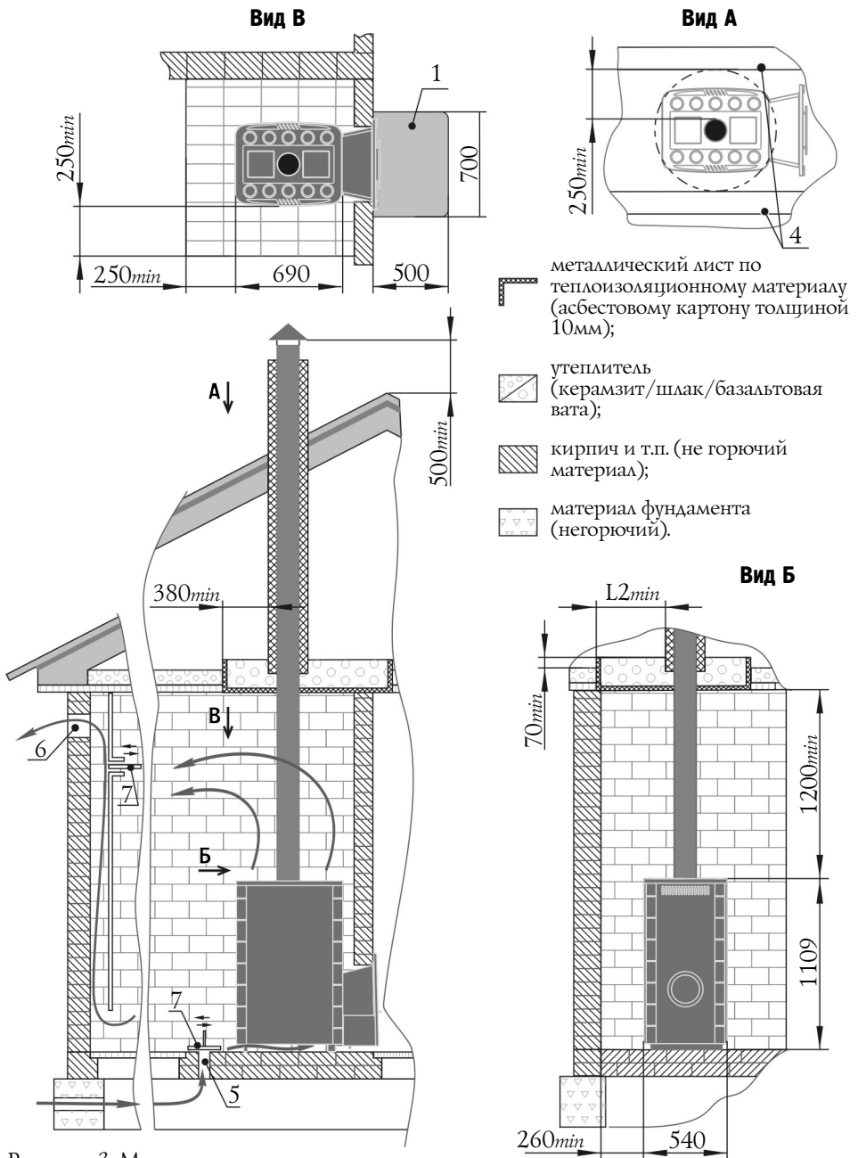
Рисунок 3. Монтаж печи с использованием кладки из негорючего материала.
