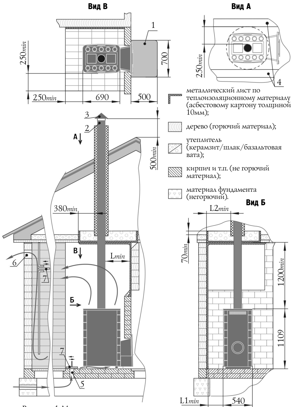
Рисунок 4. Монтаж печи с использованием кладки из негорючего материала и металлического листа по асбесту.
