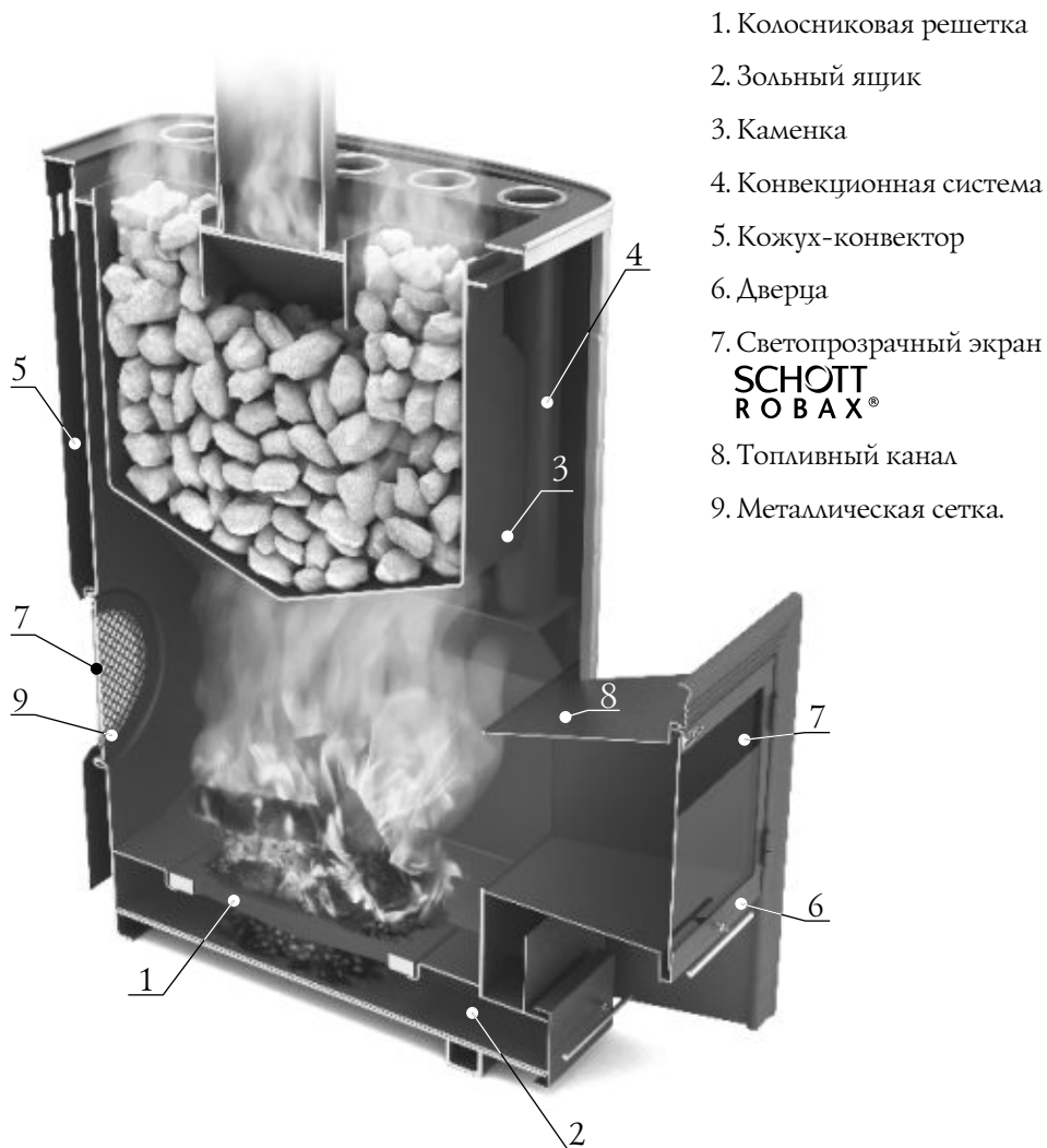
Рисунок 2. Расположение основных элементов печи ГЕКЛА.
